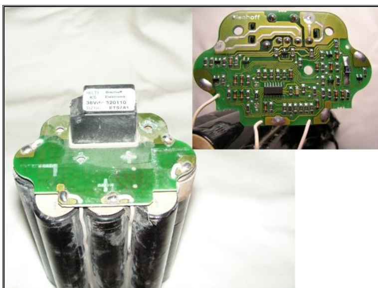
La carte électronique gérant la sécurité de décharge
